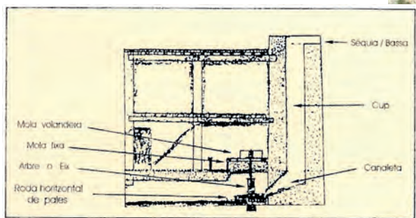
Sección del molino de Vasalo o del Turco (Dibujo de Tomás Pérez Medina).
