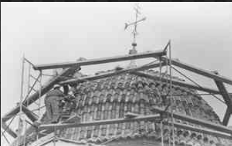
Reparación de la cúpula de la ermita de Sant Bonifaci que resultó un fracaso estético porque las tejas se "destiñeron".
