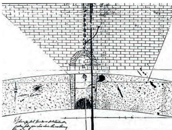
Planta y sección de la presa realizado por el maestro de cantería Chochim Bernabéu (1679).
